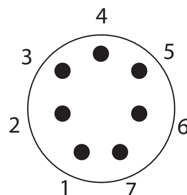
Britisch-7-Stift
