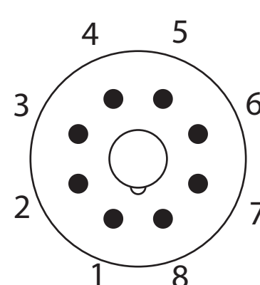
Oktal
