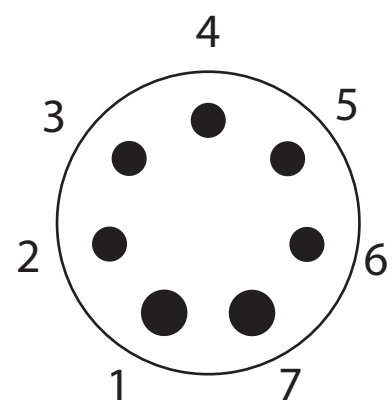
US-7-Stift (klein)
