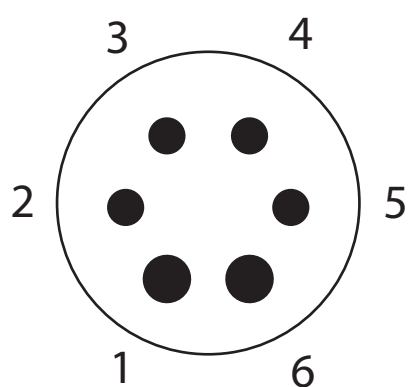
US-6-Stift (klein)
