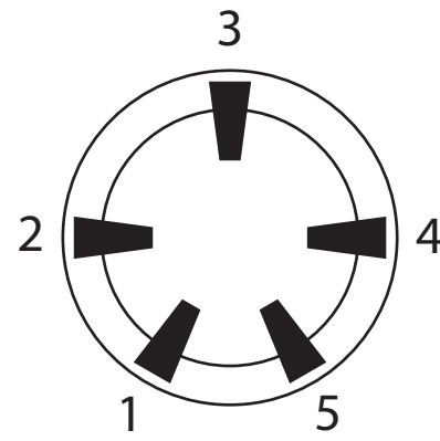
Aussenkontakt-5-Stift
