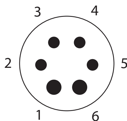
US-6-Stift (groß)
