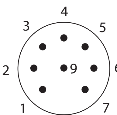
Miniatur
