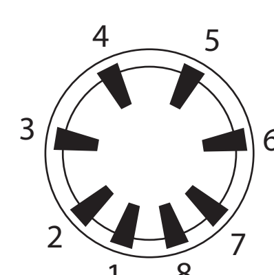
Aussenkontakt-8-Stift
