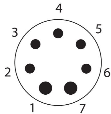
US-7-Stift (groß)
