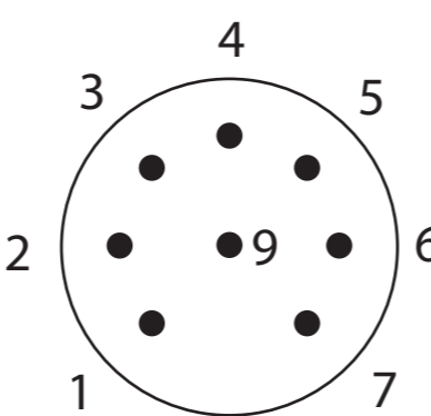
Miniatur
