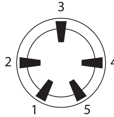
Aussenkontakt-5-Stift
