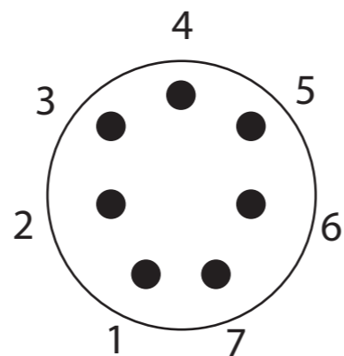
Britisch-7-Stift
