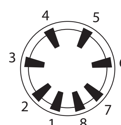
Aussenkontakt-8-Stift
