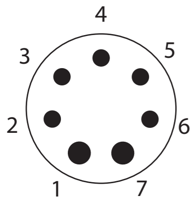
US-7-Stift (klein)
