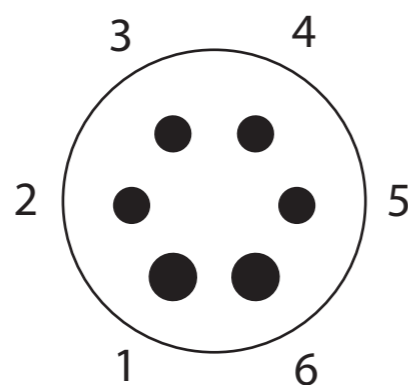
US-6-Stift (groß)
