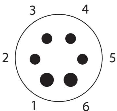
US-6-Stift (klein)
